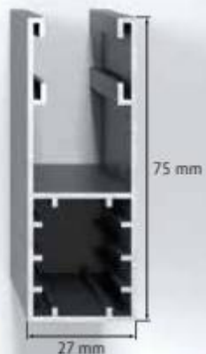
Coulisse pour Lame Isolante 55 mm Guide rail for Slats with isolation 55 mm
